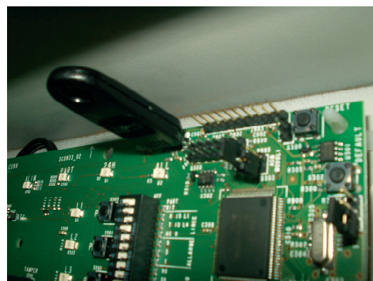
Tacca di riferimento sulla scheda di centrale
